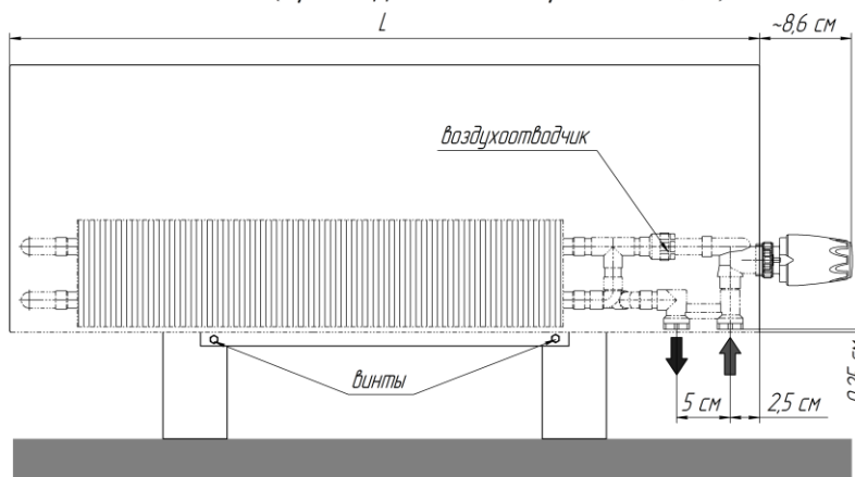
Вид для исполнения "нв" (нерегулируемая высота)
