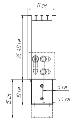
Исполнение "рв" (регулируемая высота)
