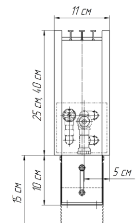
Исполнение "рв" (регулируемая высота)
