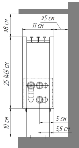
Исполнение "нв" (нерегулируемая высота)
